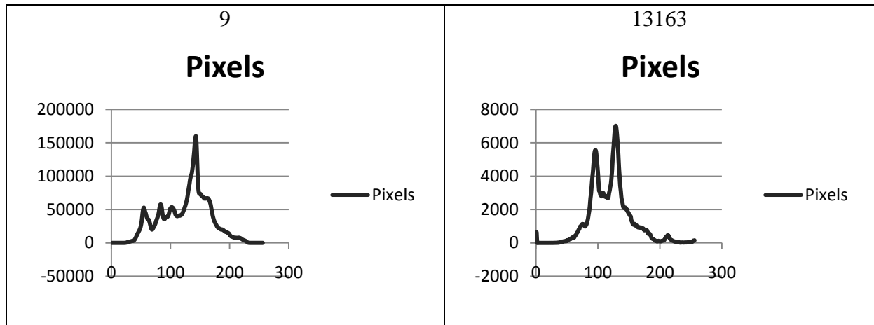
Figure A.3. Les différents graphes représentant les niveaux du contraste et de la brillance des images traitées pour évaluer l'uniformité de la distribution de la lumière au niveau de la mosquée de Bounora. (Source : Auteur)
