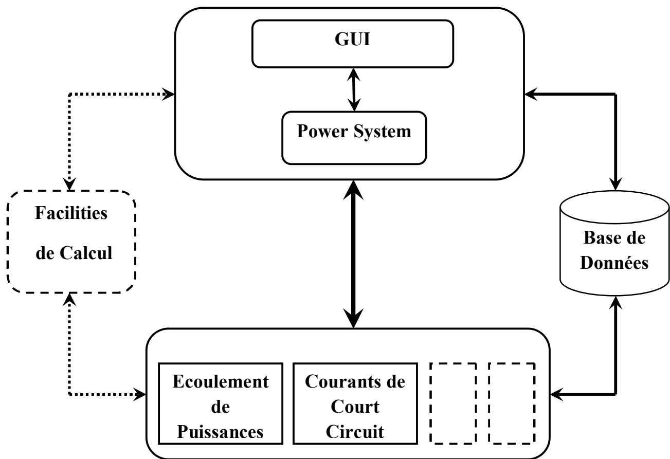
FIGURE 2.1 : Structure générale
