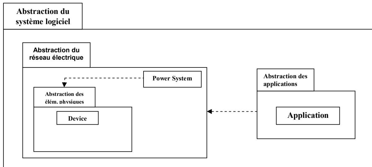
FIGURE 2.2 : Abstractions du système logiciel
